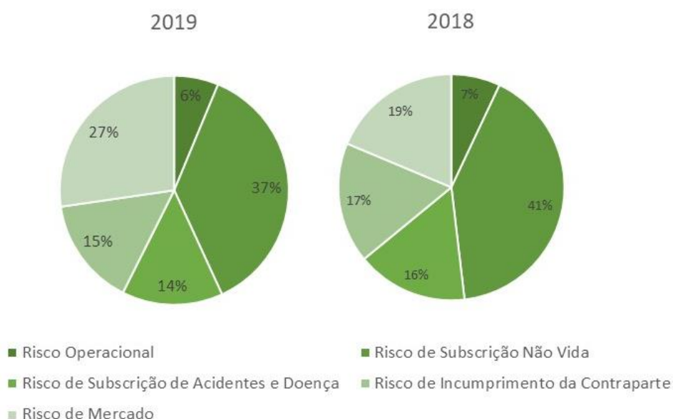
Figura 3 – Contribuição dos módulos da fórmula padrão para o SCR
